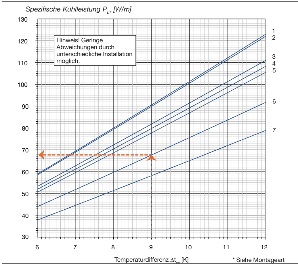
Diagramm 2. Atrium Plana, spezifische Kühlleistung P_{LT} pro aktiver Länge bei nominalem Wasserdurchfluss, q_{wnom} = 0,028 l/s.
