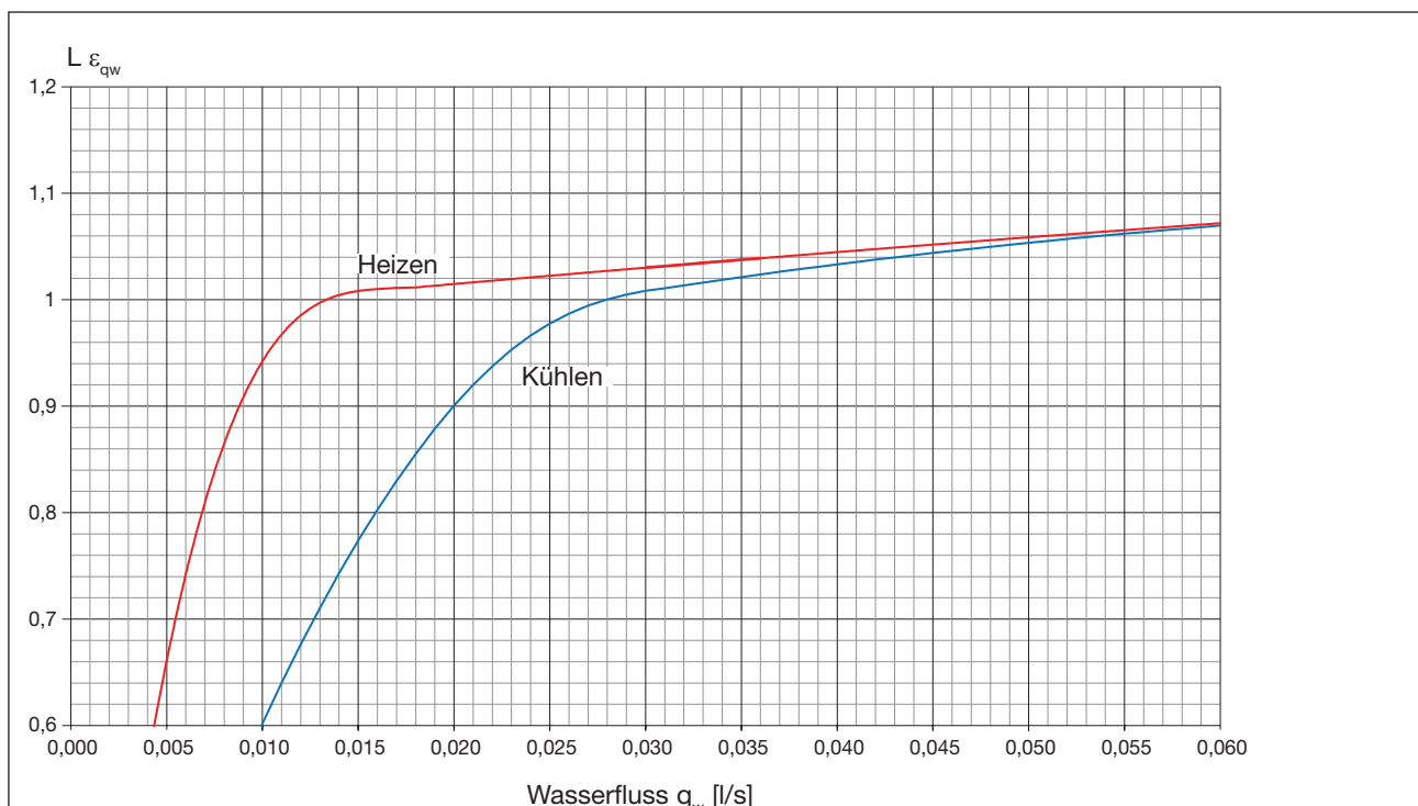
Diagramm 3. Leistungskorrektur \epsilon_{q_w} als Funktion des Wasserflusses q_w .
