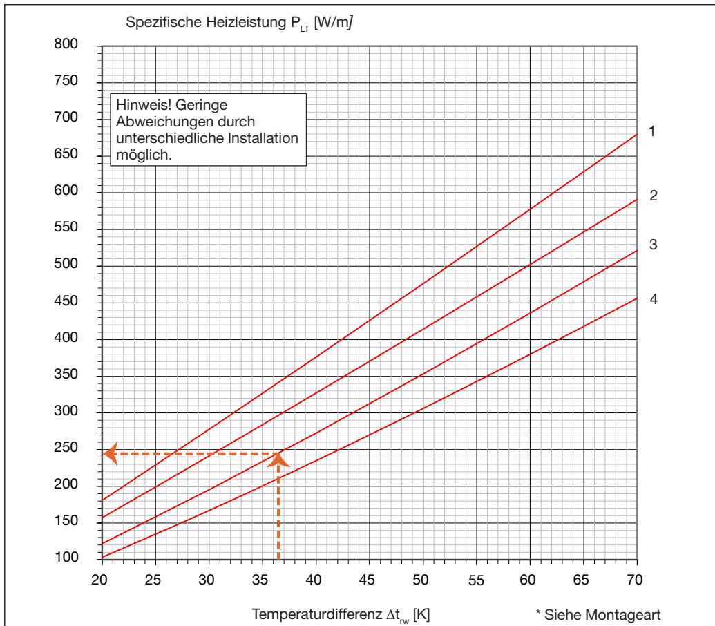
Diagramm 1. Atrium Plana, spezifische Heizleistung P_w pro aktiver Länge bei nominalem Wasserdurchfluss, q_{w, nom} = 0,0135 in Abhängigkeit von der Temperaturdifferenz \Delta t_w .
