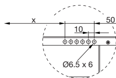
Montagevorbereitung (4 Stk. bei L_{nom} < 2,4 m und 6 Stk. bei L_{nom} \geq 2,4 m)
