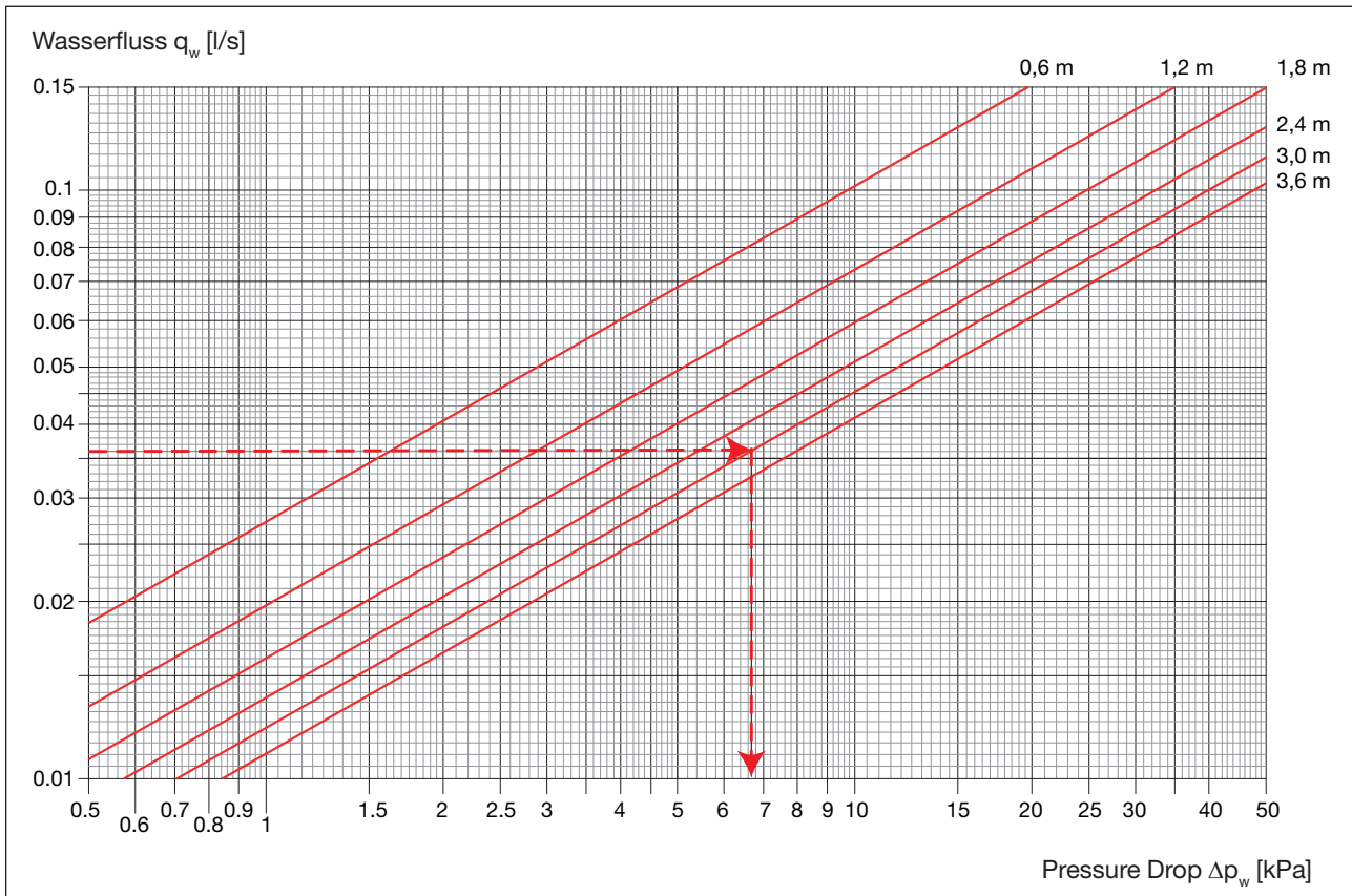
Diagramm 4. Druckverlust Atrium Plana C-60 / H-60 bei 60°C. Für Druckverluste bei anderen Temperaturen als 60°C, wird der Druckverlust mit dem Druckverlustfaktor multipliziert (siehe Diagramm 5).
