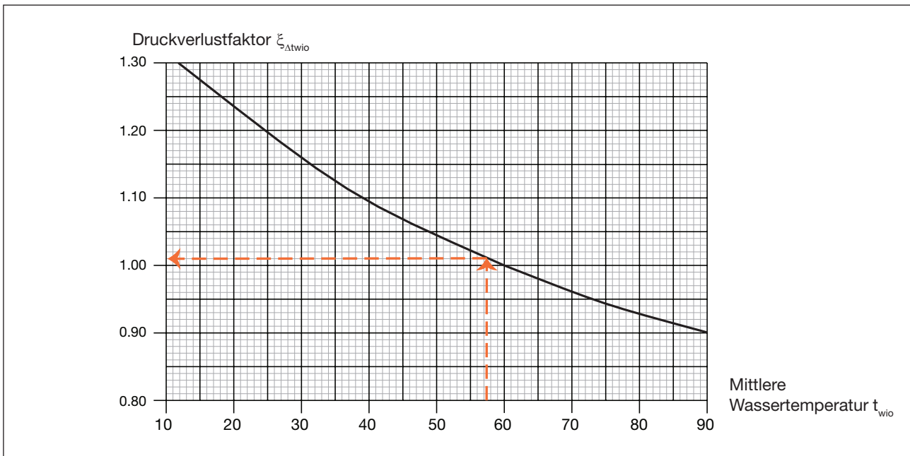
Diagramm 5. Temperaturabhängiger Druckverlustfaktor.
