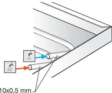
C7: Anschlussstyp 7: 15° biege
