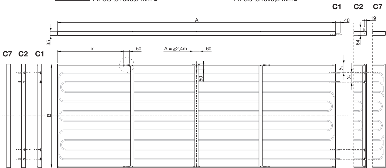
Abmessungen Kühl- und Heizpaneel.
