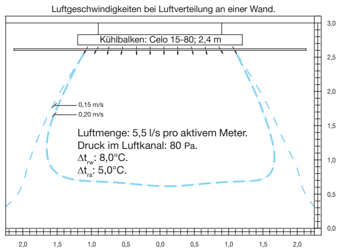
Abbildung 11 - 14: Luftgeschwindigkeiten bei Montage über der Zwischendecke; Schlitze entlang der Wand.
