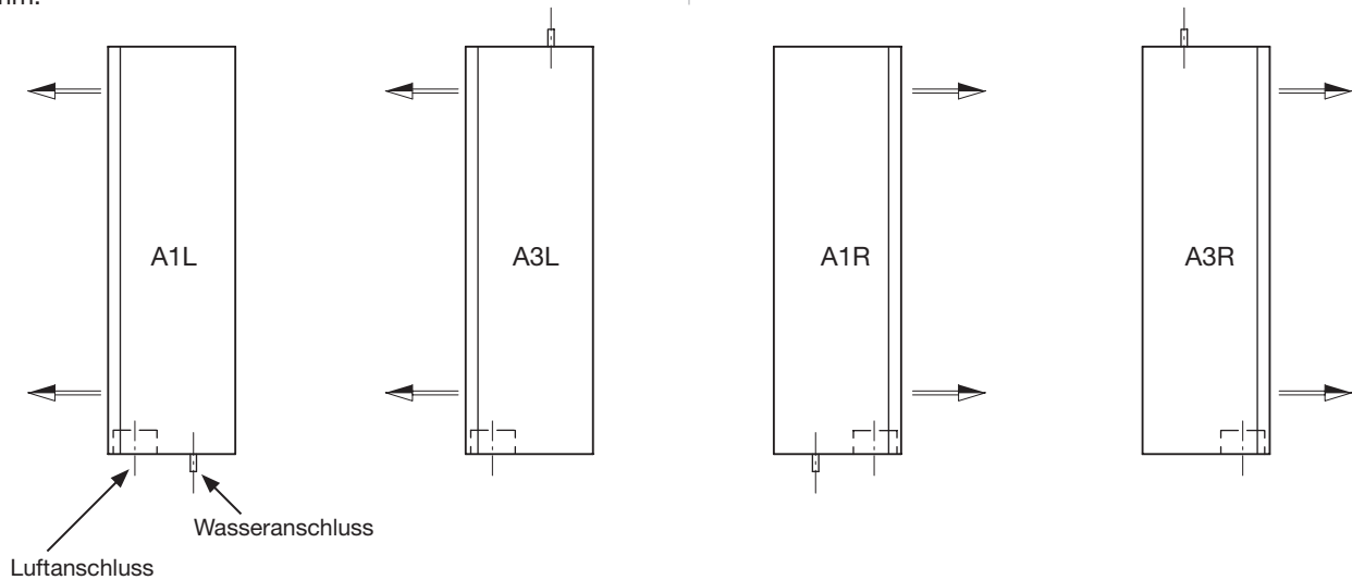
Abbildung 2: Celo hat vier verschiedene Anschlussmöglichkeiten: A1L, A3L, A1R und A3R.
