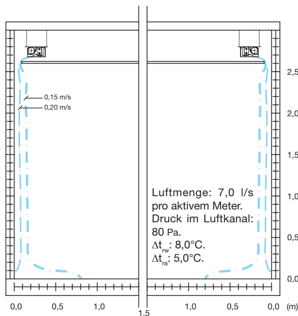
Abbildung 11 - 14: Luftgeschwindigkeiten bei Montage über der Zwischendecke; Schlitze entlang der Wand.
