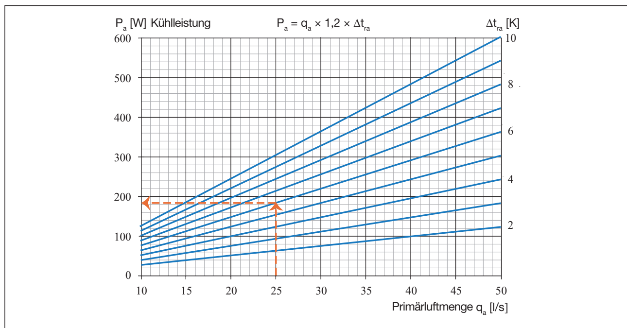
Diagramm 1. Kühlleistung P_a als Funktion von der Luftmenge q_a . Wenn die Luftmenge 25 l/s beträgt und die Temperaturdifferenz der Zuluft \Delta t_{ra} bei 6 K, liegt die Kühlleistung entsprechend dem Diagramm bei 180 W.
