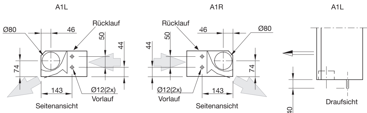
Abbildung 3: Abmessungen der Anschlüsse beim Celo.
