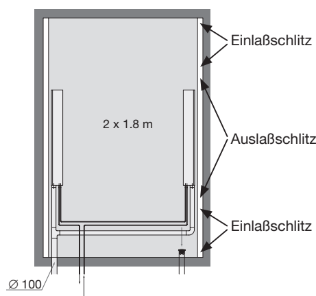
Abbildung 1: Zwei Celo Balken mit offenen Schlitzen.
