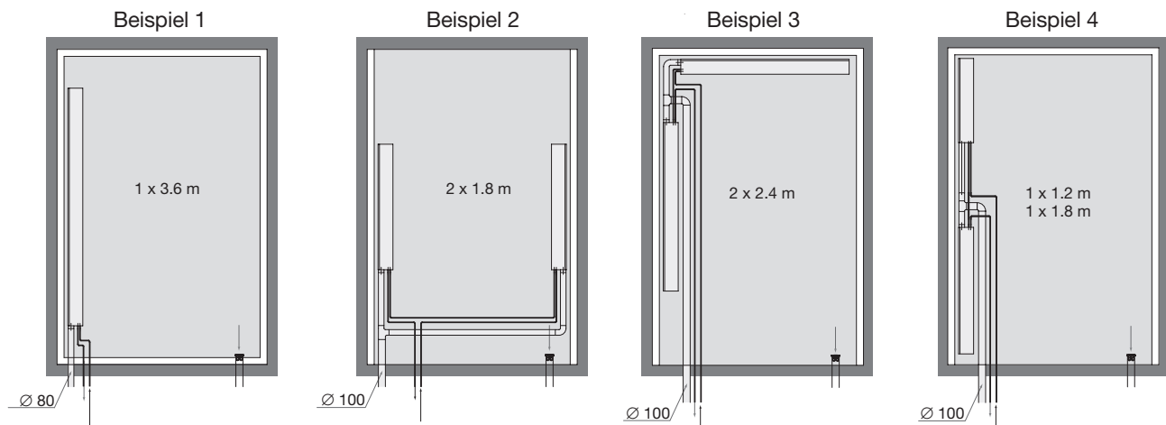
Abbildung 9: Vier Beispiele wie Celo in Kombination mit verschiedenen Schlitten in der Zwischendecke inklusive passendem Luft- und Wasseranschluss montiert werden kann.
