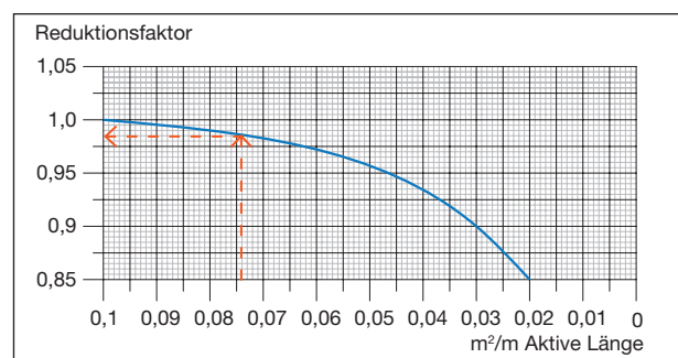
Diagramm 5: Leistungsreduktion aufgrund von reduziertem Einsaugschlitz.
