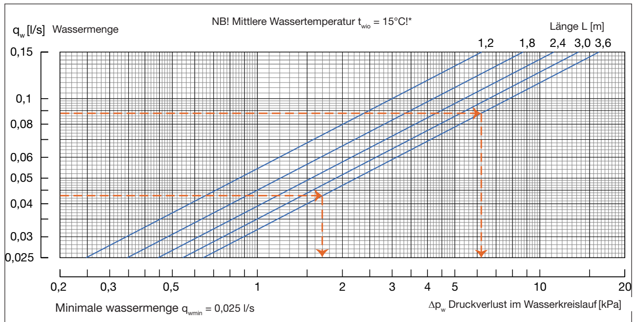
Diagramm 4: Druckverlust im Wasserkreislauf, Kühlung.
