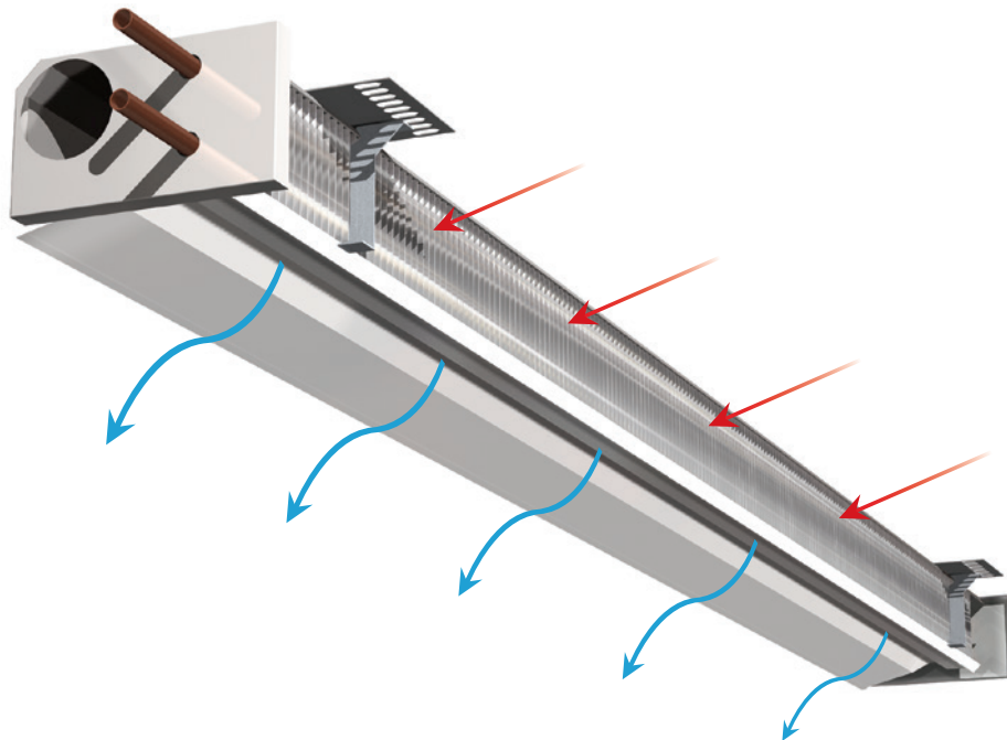
Bild 1: Celo arbeitet nach dem Induktionsprinzip.
