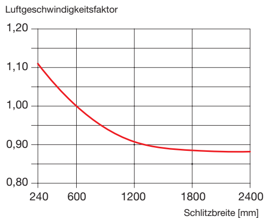
Abbildung 15 - 18: Luftgeschwindigkeiten bei Inselmontage.
