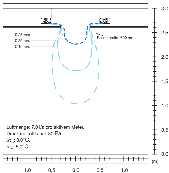
Abbildung 15 - 18: Luftgeschwindigkeiten bei Inselmontage.
