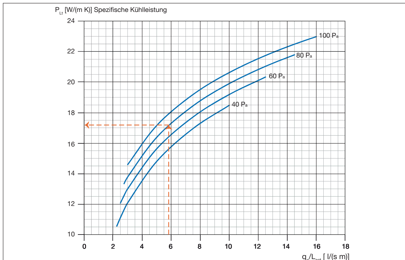
Diagramm 2: Spezifische Kühlleistung P_{Lt} pro aktiven Meter und Kelvin als Funktion von Luftmenge pro aktiven Meter bei Düsendruck von 40, 60, 80 und 100 Pa.
