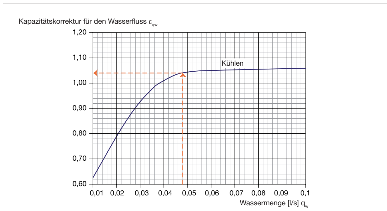
Diagramm 3: Kapazitätskorrektur für den Wasserfluss \varepsilon_{qw}
