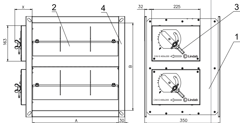
Volumenstromregler - manuelle Verstellung - B \geq 400 mm
