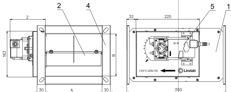
Volumenstromregler - motorische Verstellung
