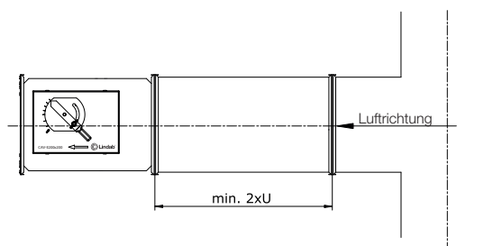
Empfohlener Abstand zu einem Abzweig
