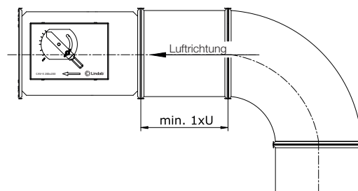
Empfohlener Abstand zu einem Bogen
